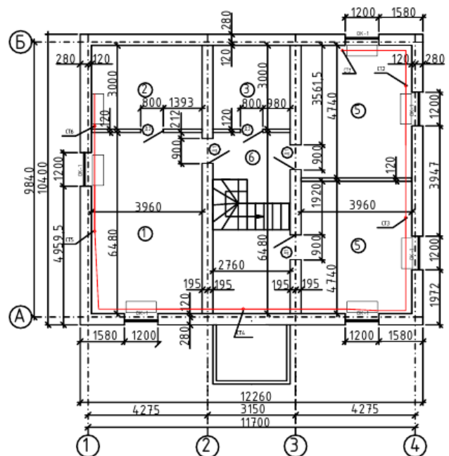
План 2 этажа
